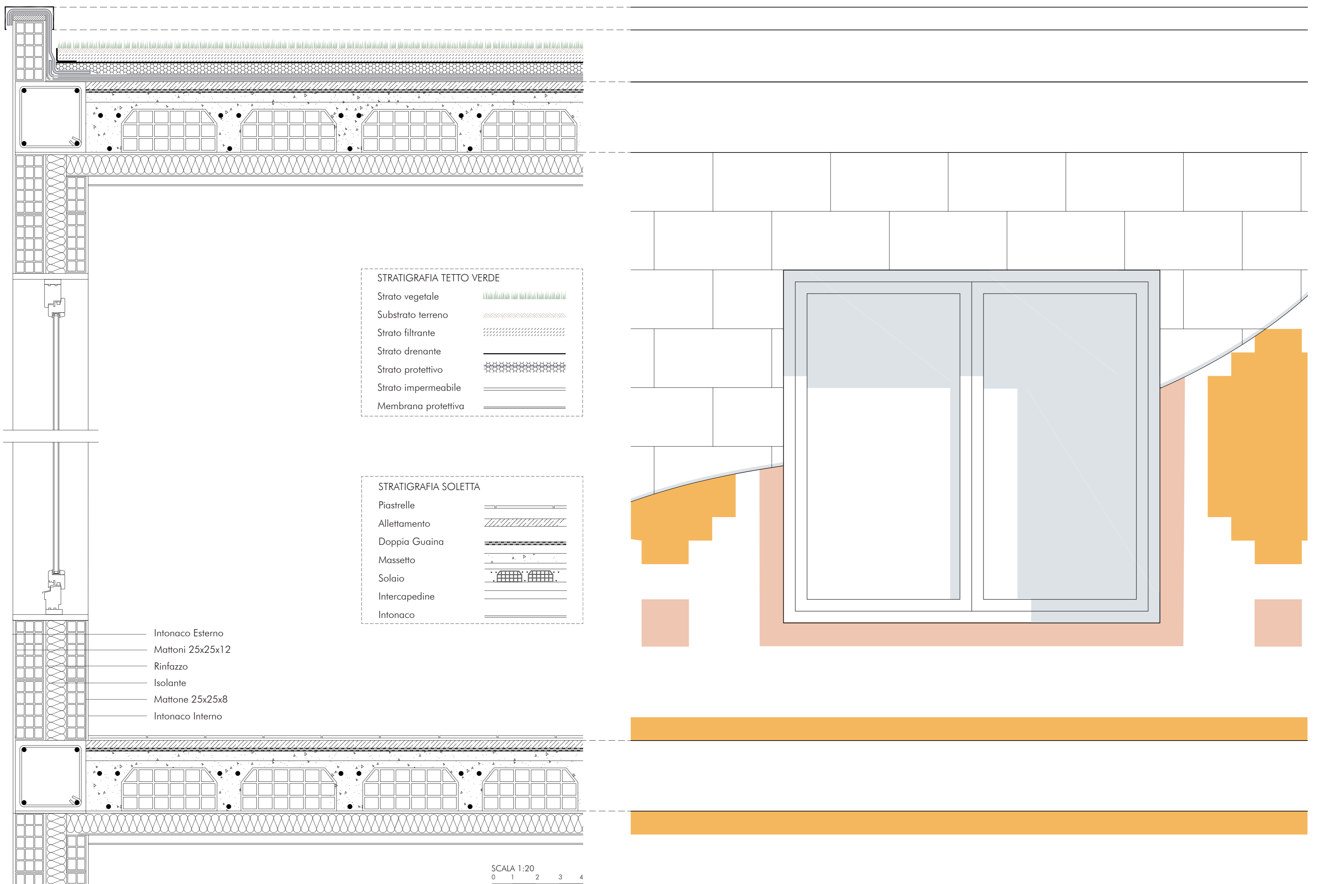
DETTAGLIO COSTRUTTIVO, TETTO VERDE E SOLAIO
