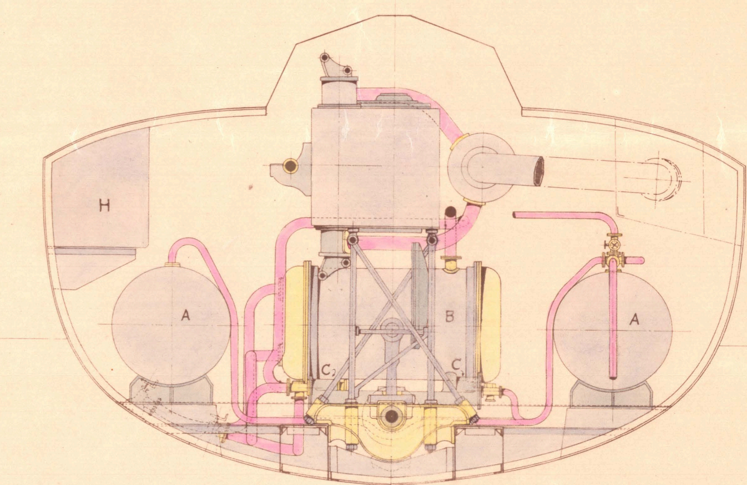
SEZIONE SULL'ORDINATA 48.
