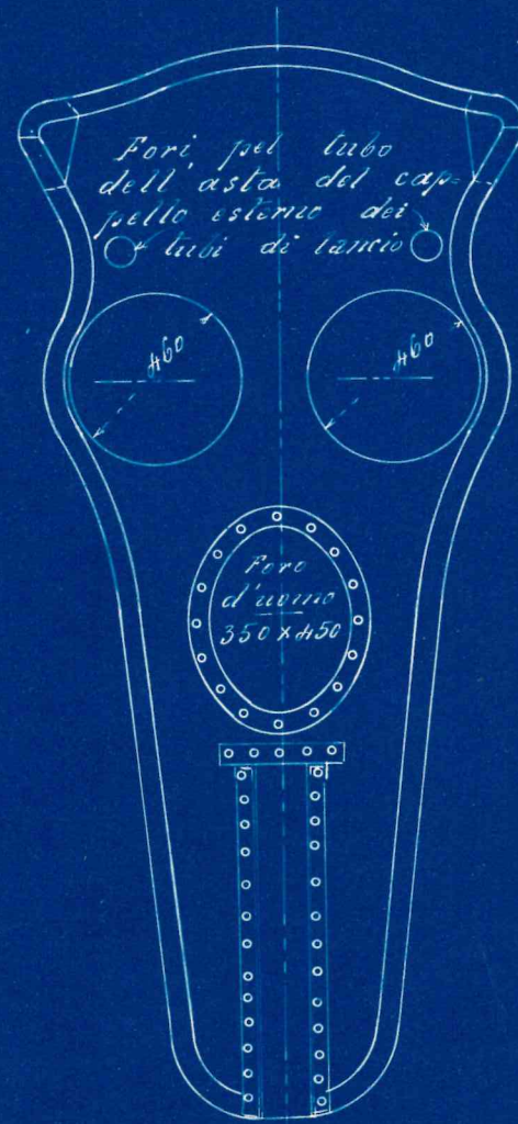
Paratia stagna Ord. n° 5. vista da poppa
