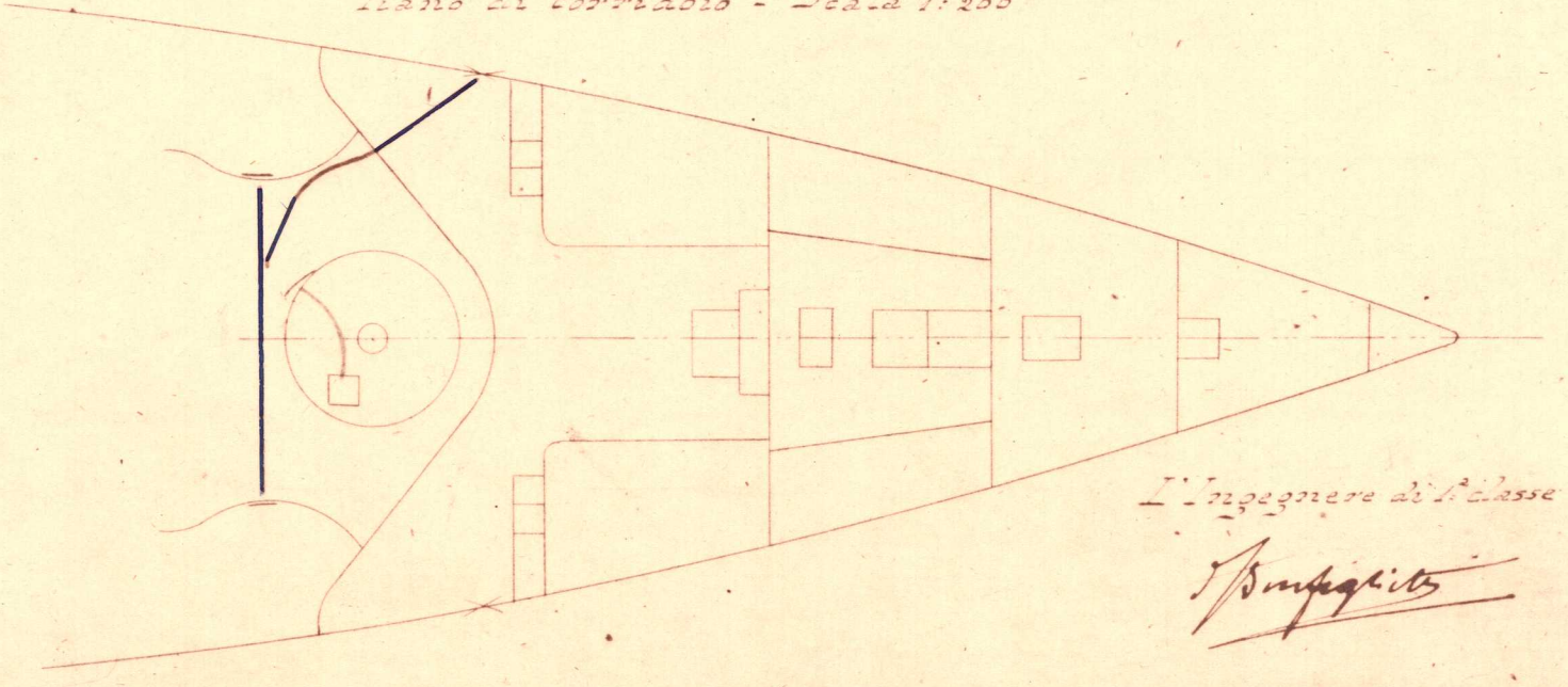
Piano di corridoio - Scala 1:200
