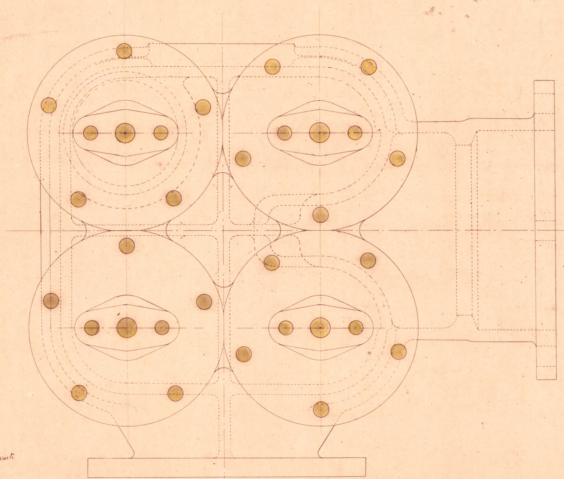
Gruppo di valvole per l'esarimetro del doppio fondo. Scala 1/2
