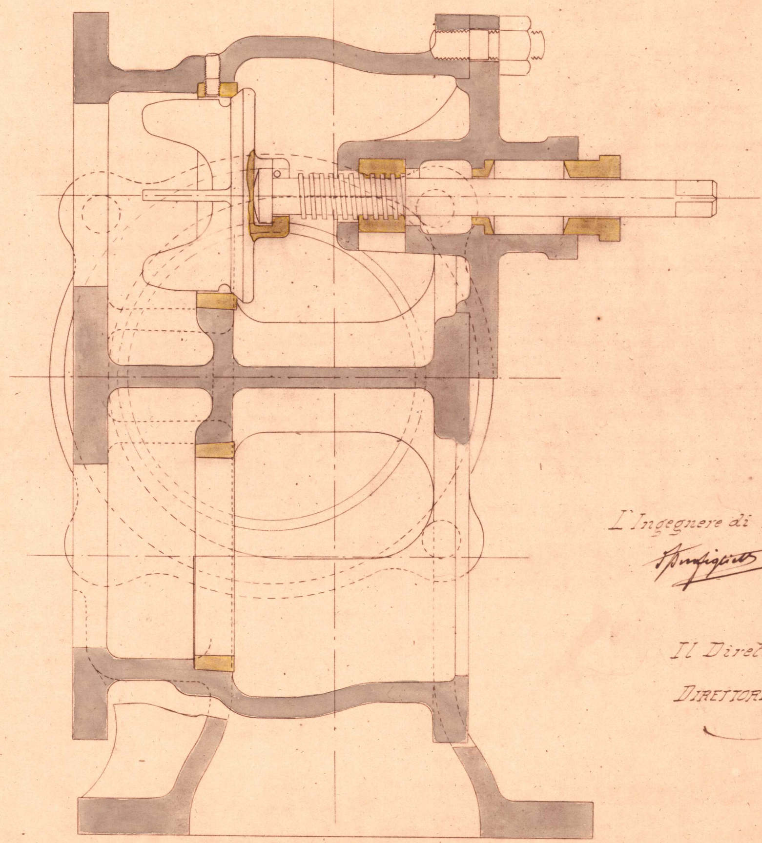
Gruppo di valvole per l'esarimetro del doppio fondo. Scala 1/2
