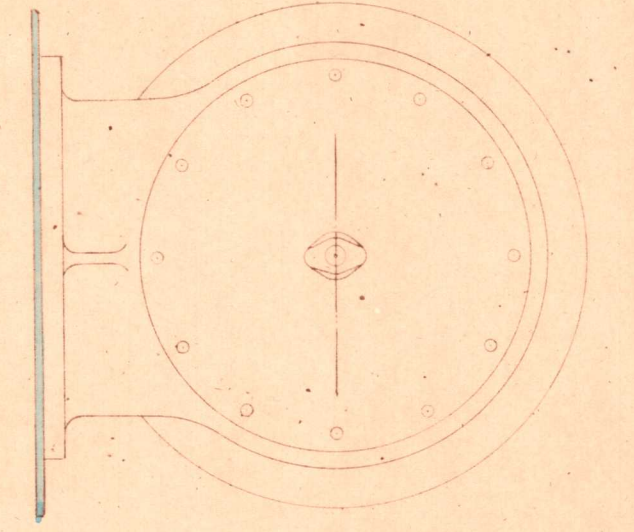
Tipo di valvola per il grande esaurimento - Scala \frac{1}{10}
