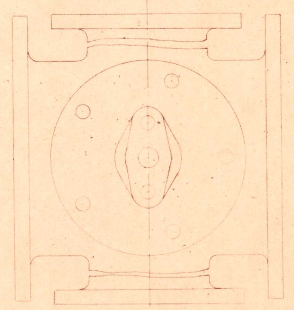
Tipo di valvola per l'esaurimento delle sentine Scala \frac{1}{4}
