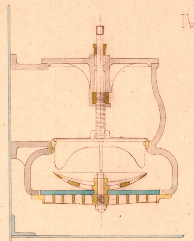
Tipo di valvola per il grande esaurimento - Scala \frac{1}{10}
