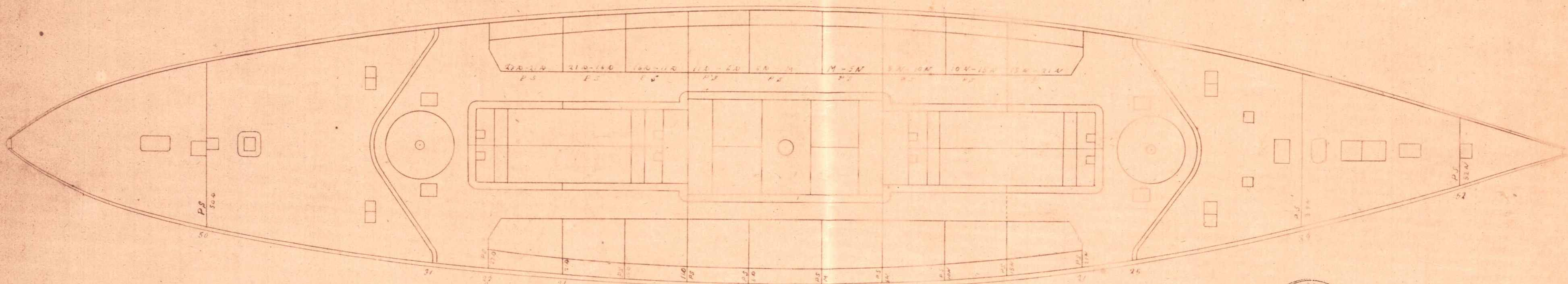
PONTE DI PROTEZIONE
